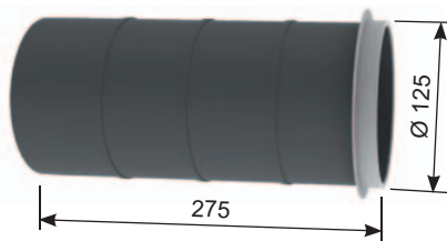
Manchon traversée de dalle
