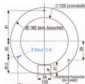
Schéma platine
