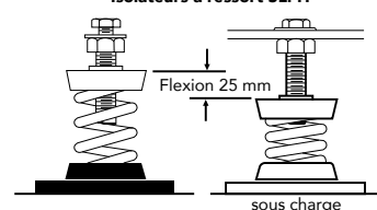
Isolateurs à ressort SLFH
