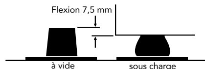
Isolateurs en néoprène ND
