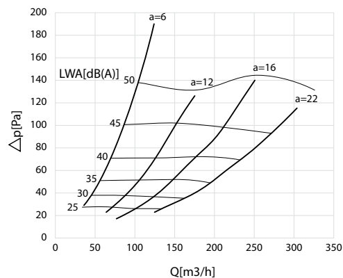
amenée d'air
