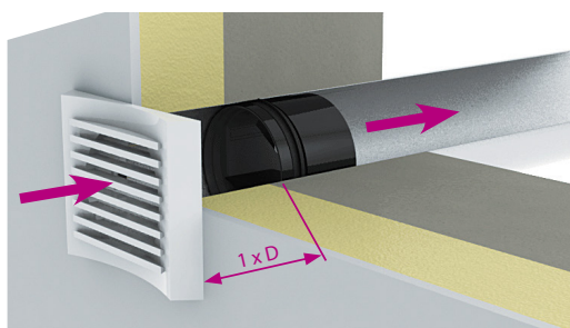
Régulateur RD en extraction
