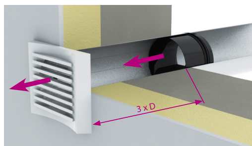
Régulateur RD en soufflage
