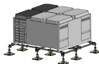
Conception en treilli pour une unité surdimensionnée
