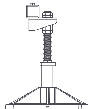
Ensemble de pied standard Hauteur réglable: 335 - 440 mm
