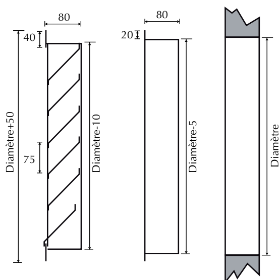
EXT-C pas de 75 mm
