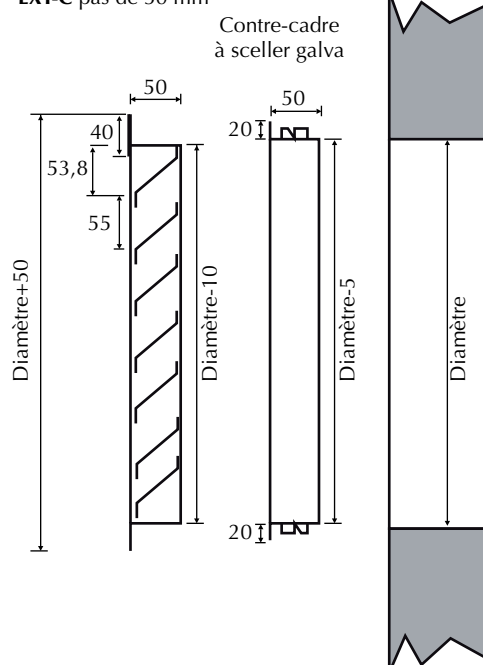
EXT-C pas de 50 mm
