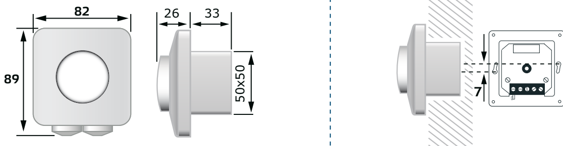
Fig. 2 Dimensions de montage – montage encastré
