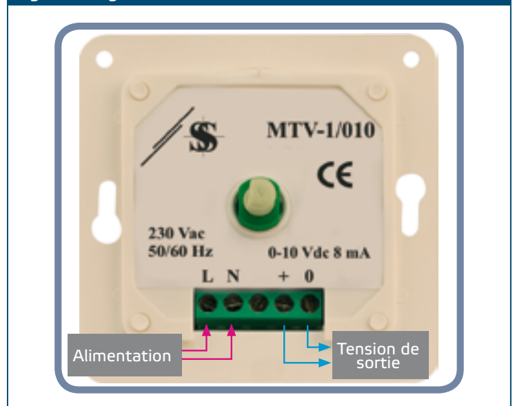
Fig. 1 Câblage et raccordements
