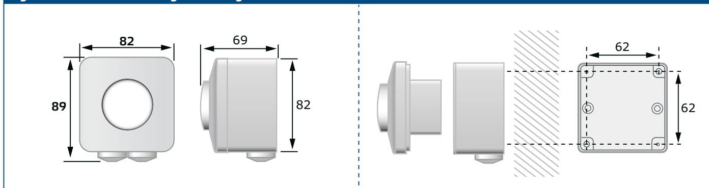
Fig. 3 Dimensions de montage – montage en surface
